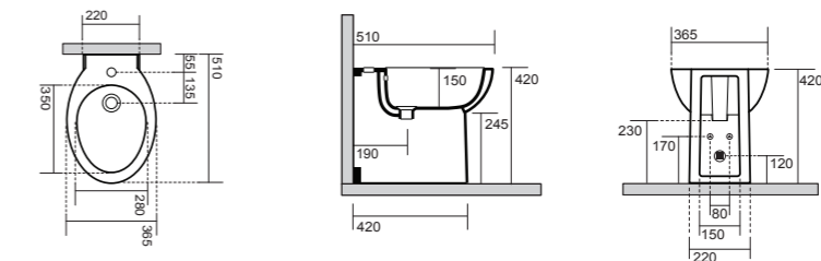
Bidet Terra BTW Bidet 36,5x51 cm
