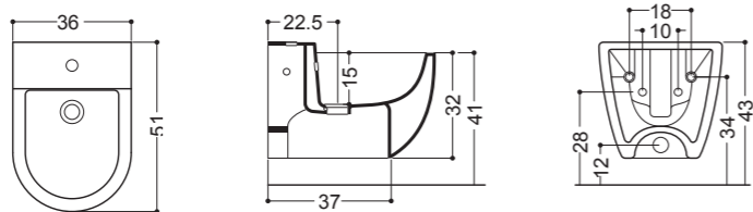
Bidet Sospeso Wall-hung Bidet 36x51 cm
