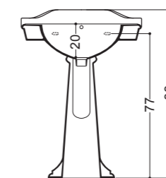
Lavabo angolare Corner Basin 60x48 cm
