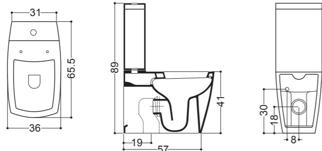
Vaso Monoblocco BTW Monobloc Wc 36x65,5 cm
