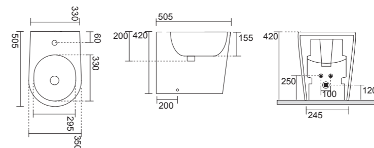
Bidet Terra BTW Bidet 33x50 cm
