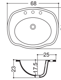
Lavabo incasso Inset Basin 68x54 cm
