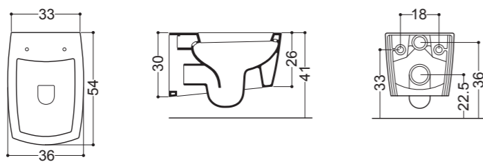
Vaso Sospeso Wall-hung Wc 36x54 cm
