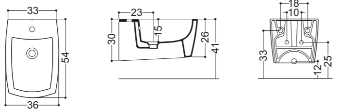
Bidet Sospeso Wall-hung Bidet 36x54 cm
