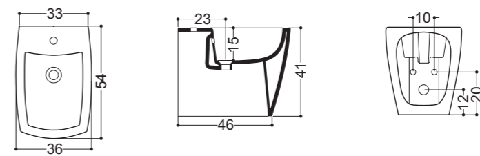
Bidet Terra BTW Bidet 36x54 cm
