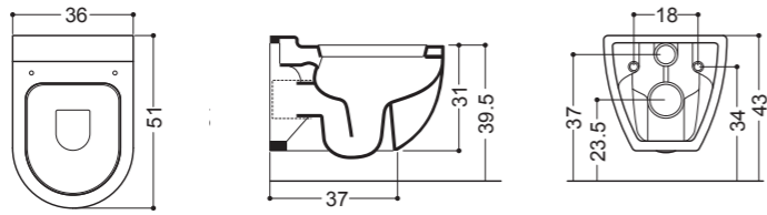
Vaso Sospeso Wall-hung Wc 36x51 cm
