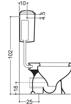
Art 06052 Cassetta Zaino Low level cistern 38x45,5 cm
